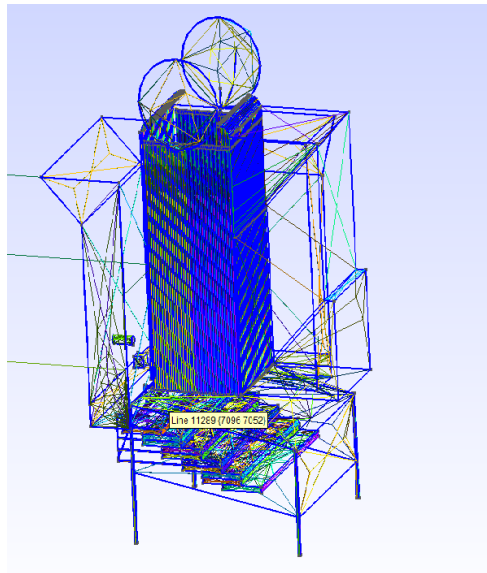
Gmsh التشبيك للتصميم عبر: Figure 11.1.3-6:
