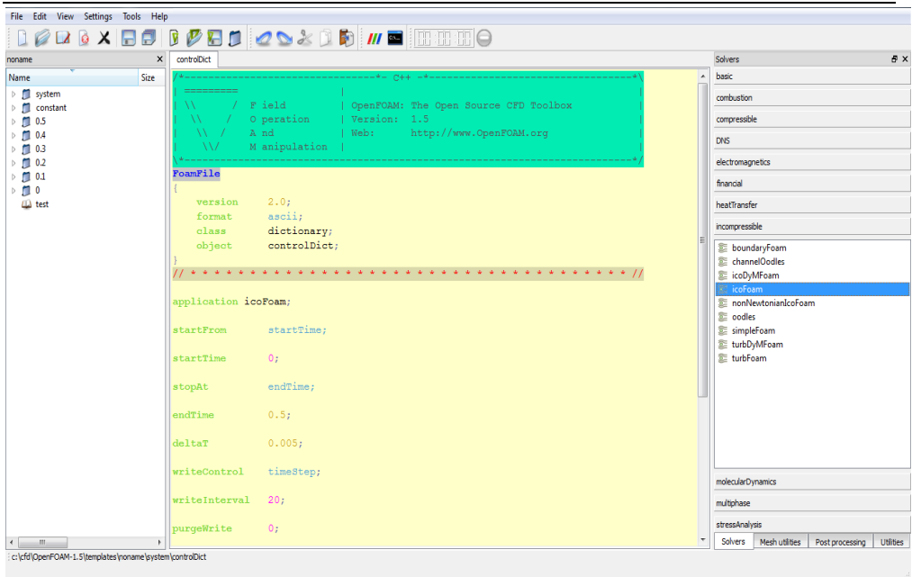
Figure 11.2.1-10:2 OpenFOAM نتائج في windows
