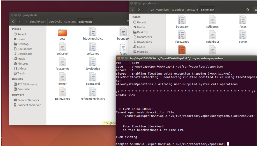
Figure 11.1.3-7: واجهة Linux-Ubuntu
